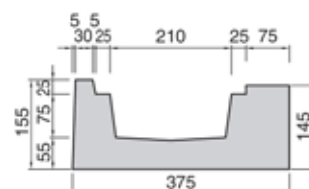
Sezione
