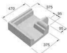
Sezione Angolo Retto
