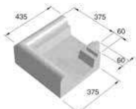
Sezione Angolo Retto Rovescio
