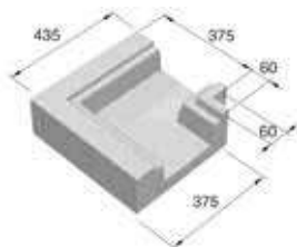
Sezione Angolo Retto Rovescio
