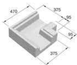
Sezione Angolo Retto
